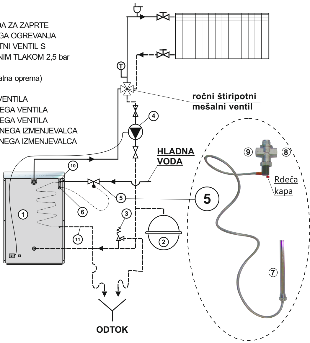
Shema 2. - Priključitev kotla BIO-CET 17 B
